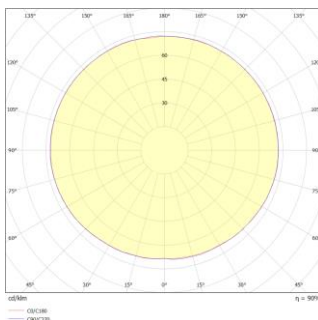
Ø 60 cm
